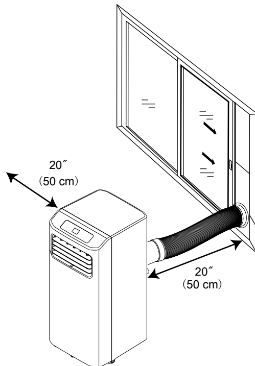
Instalación en ventana corrediza horizontal
