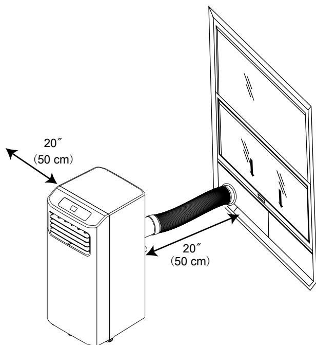
Instalación en ventana corrediza vertical
