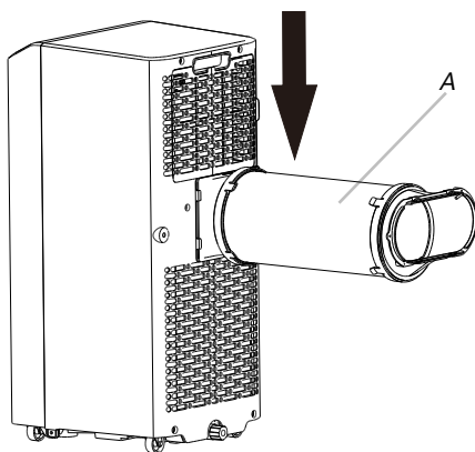
A. Manguera de escape flexible
