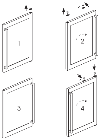
Parte superior del agujero del eje izquierdo Parte superior del agujero del eje derecho (como se suministra)
